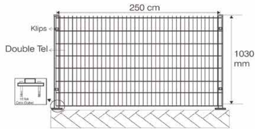
Double panel çit uygulama
